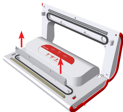
Slika 6: Če tekočina zaide v vakuumski kanal, dvignite posodico naravnost navzgor, izlijte tekočino in posodico dobro osušite.
