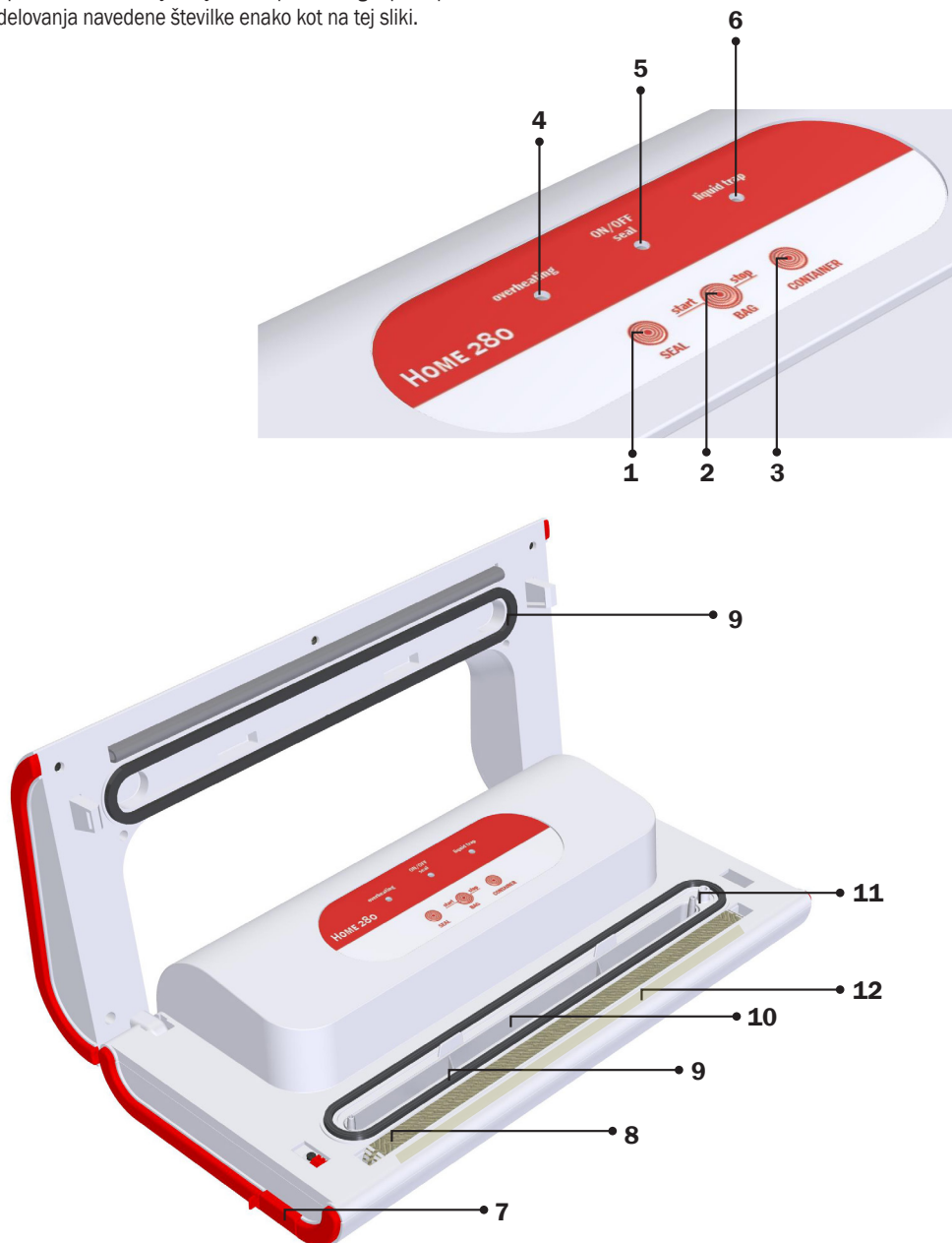
Slika 1: Status Home 280 z označenimi sestavnimi deli.
