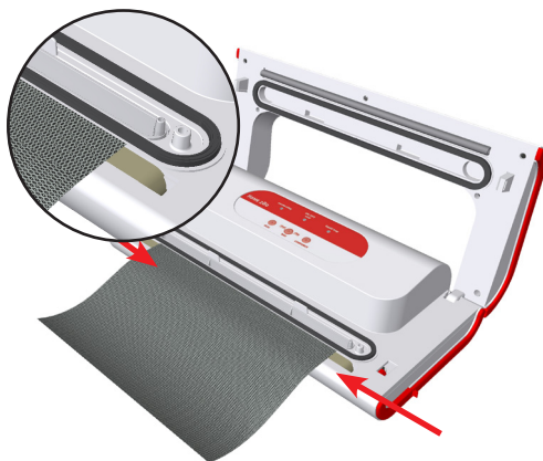
Slika 4: Pri varjenju nastavite vrečko preko varilnega traku do črnega tesnila.
