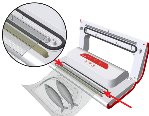
Slika 5: Pri vakuumiranju namestite odprti rob vrečke v sredino vakuumskega kanala.
